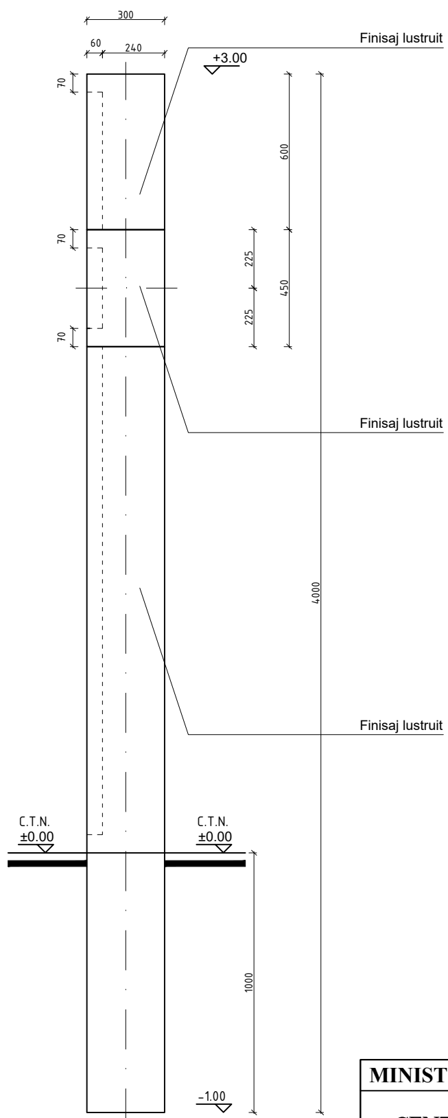
VEDERE LATERALĂ STÂNGA/DREAPTA CRUCE MARMURĂ SCARA 1 : 20 - cote în mm
