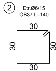
SECTIUNE 1-1 SCARA 1 : 20
