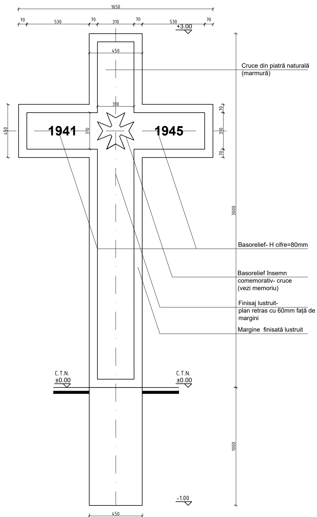
VEDERE FRONTALĂ CRUCE MARMURĂ SCARA 1 : 20 - cote în mm
