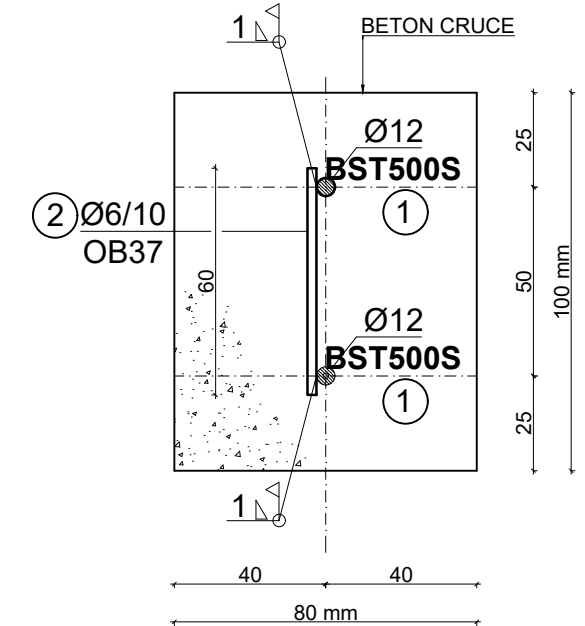
SECTIUNE b - b SCARA 1 : 5
