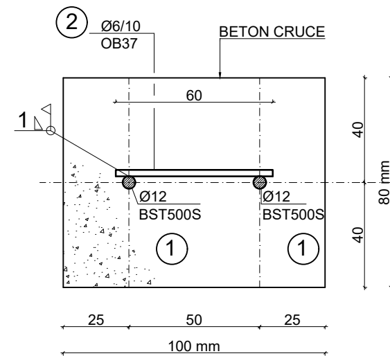
SECTIUNE a - a SCARA 1 : 5
